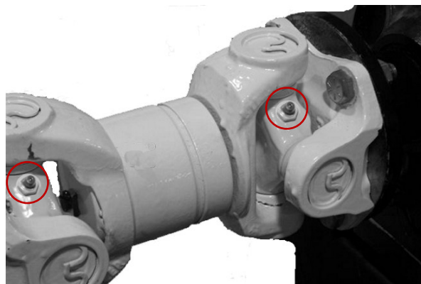
Joint de cardan d'arbre moteur avec graisseurs
