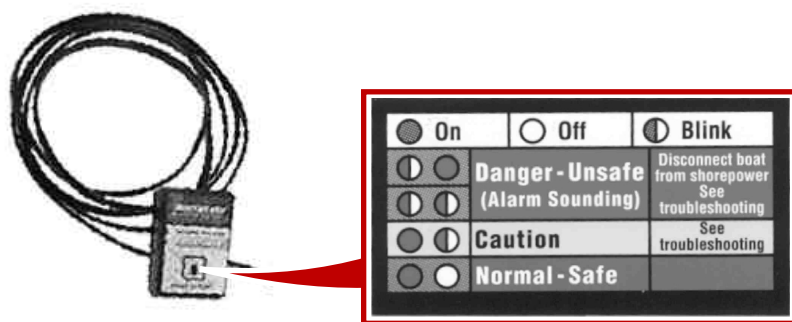
Moniteur de l'isolateur galvanique et conditions
